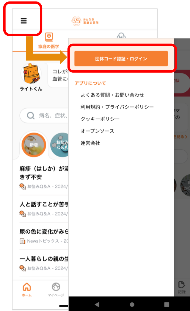
トップ画面
